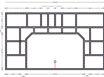
ESQUEMA DE FUNDAMENTACIÓN E. 1/200
